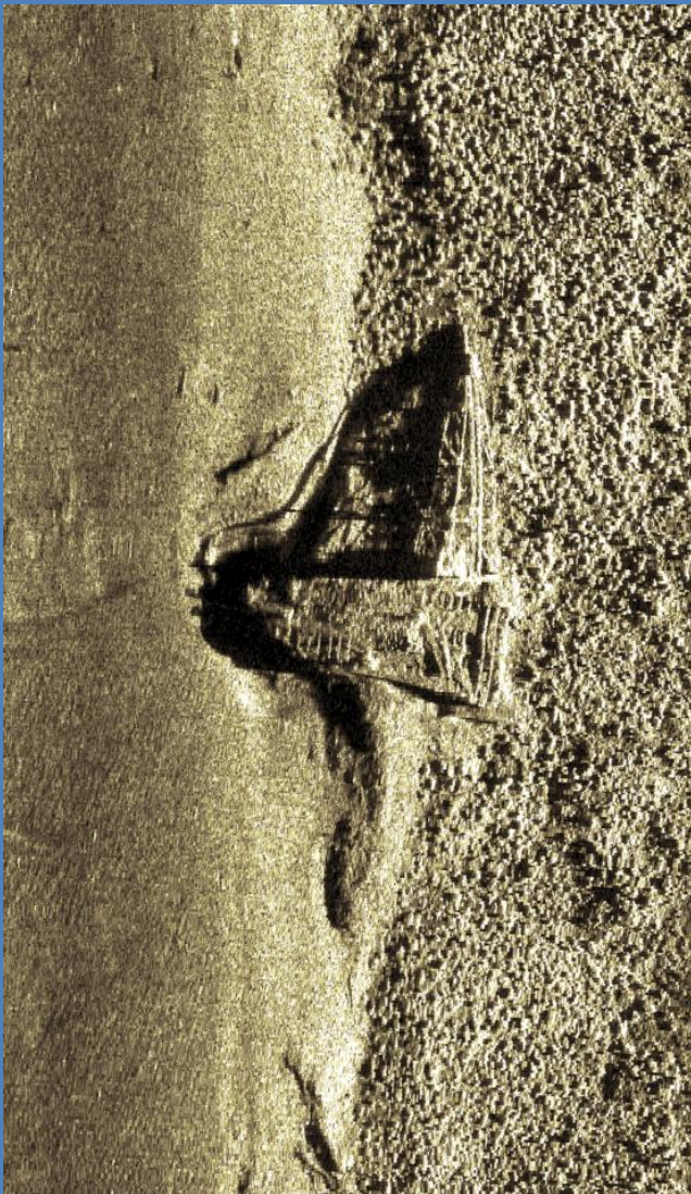
Sonar EdgeTech 4125 (600 kHz, zakres 50 m)
