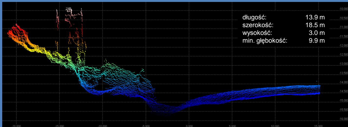
Echosonda wielowiązkowa Reson Seabat T-20P (400 kHz, 512 wiązek, 20 Hz)
