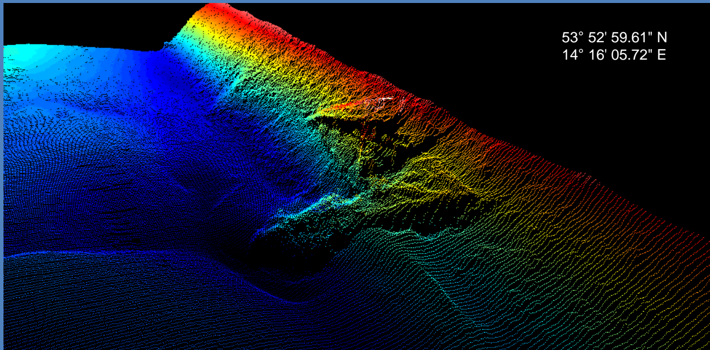
Echosonda wielowiązkowa Reson Seabat T-20P (400 kHz, 512 wiązek, 20 Hz)
