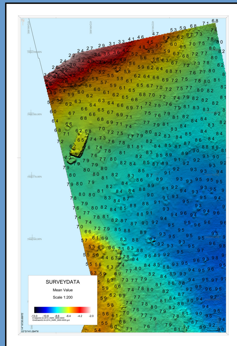
Echosonda wielowiązkowa: Reson Seabat T-20P (420 kHz, 512 wiązek, 20 Hz)
